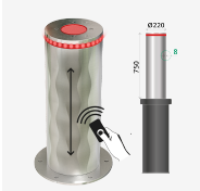
RAMBLA Ø220x750 H7508R
